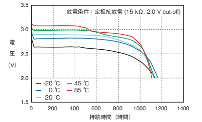
■ 放電温度特性 (CR2032Aの例)
