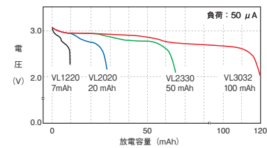
■ 放電特性の例
