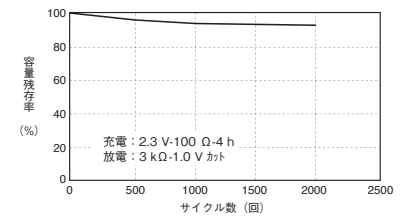
■ 充放電サイクル特性 (MT920の例)
