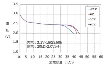
■ 放電特性
