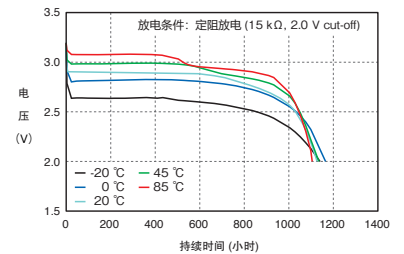
■ 放电温度特性(CR2032A示例)
