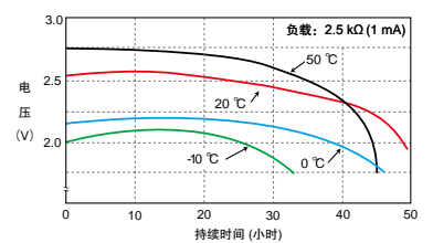
■ 放电温度特性 (BR435示例)
